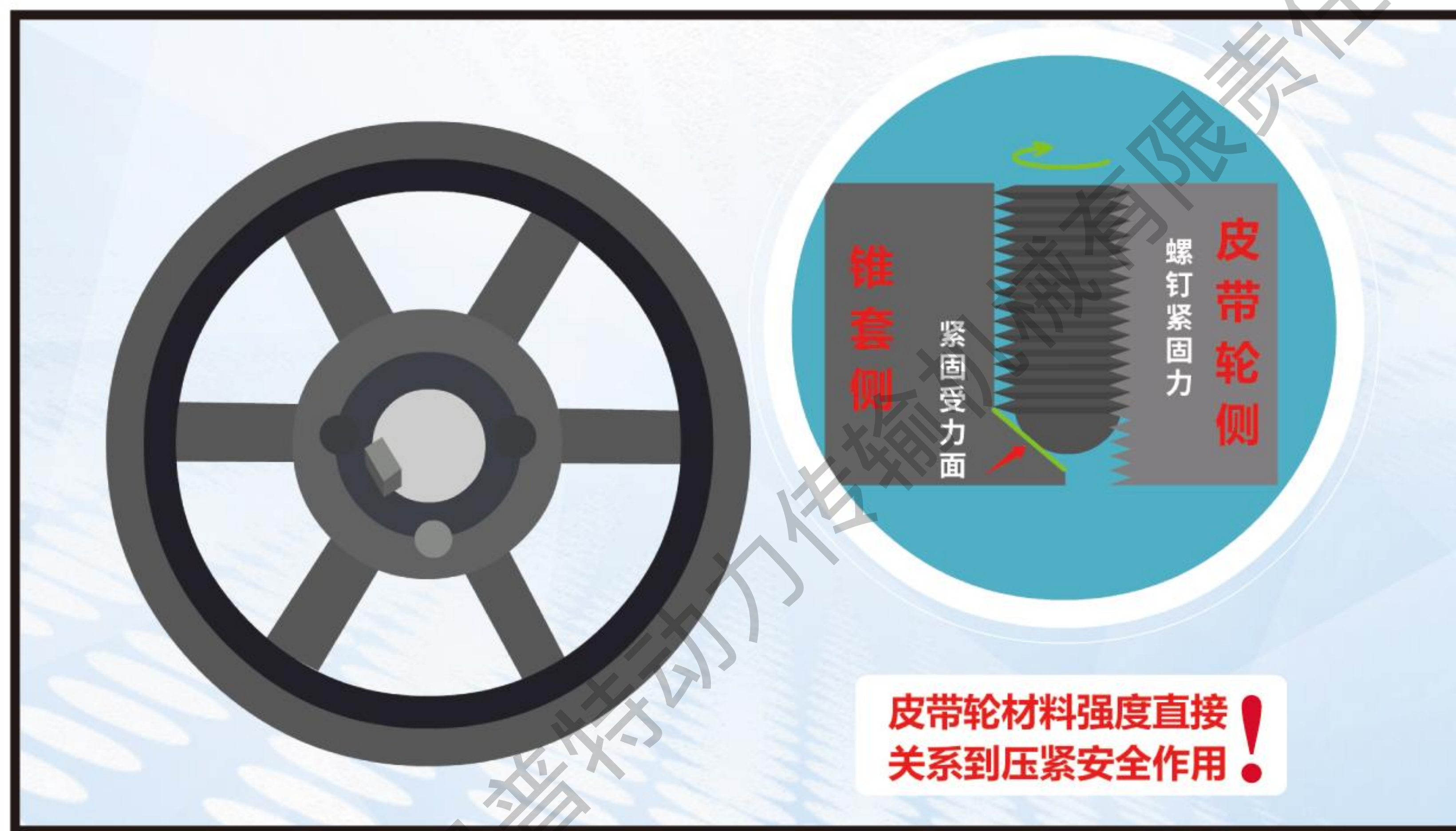
⑬ 锥套和皮带轮因拧紧力不足导致压紧失效
